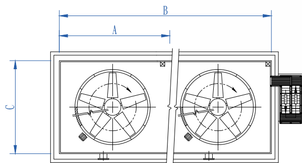
俯視圖 PLAN VIEW
