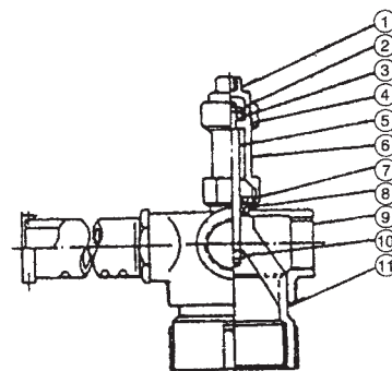
圖5 KST-N-70~1500RT
