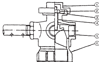
圖4 KST-N-3~60RT
